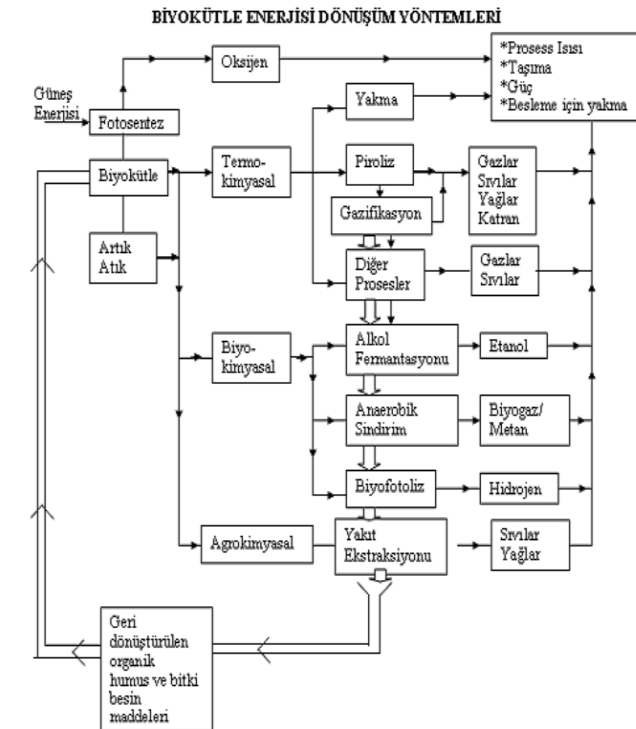
Şekil 110: Biyokütle Enerjisi Dönüşüm Yöntemleri
